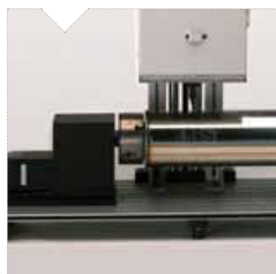
AR1 asse rotante con mandrino, portata massima 5 Kg diametro 70 mm
